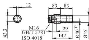
GKA/GKAZ/GKAF57输出轴
