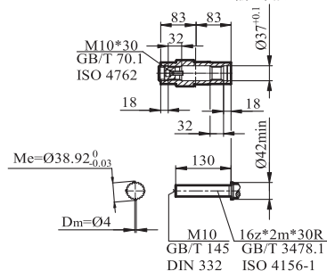
GKV/GKVZ/GKVF57输出轴
