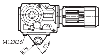
GKA/GKAZ/GKAF57输出轴
