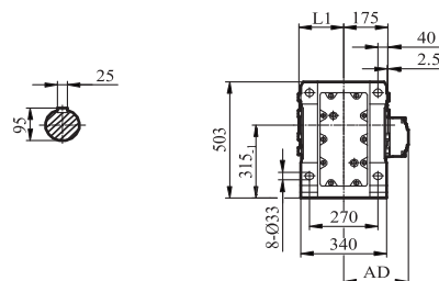
GKAZ/GKHZ/GKVZ107
