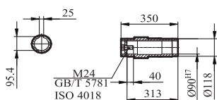
GKA/GKAZ/GKAF107输出轴
