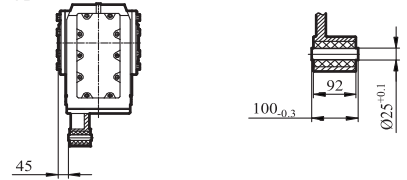
GKV/GKVZ/GKVF107输出轴
