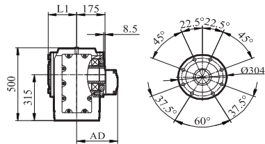
GKAZ/GKHZ/GKVZ107
