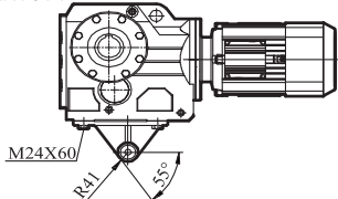
GKA/GKAZ/GKAF107输出轴
