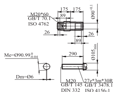
GKV/GKVZ/GKVF107输出轴
